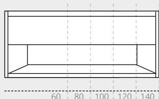
Onderkast 1 lade met open schap en inliggend front 60 / 80 / 100 / 120 / 140 x 46 x 52 cm
