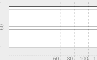
Onderkast 2 laden symmetrisch met opliggende fronten 60 / 80 / 100 / 120 x 46 x 52 cm
