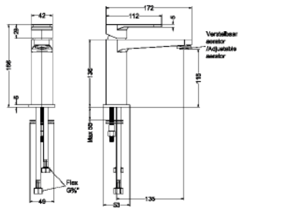
Wastafelmengkraan staand model S - Forma
