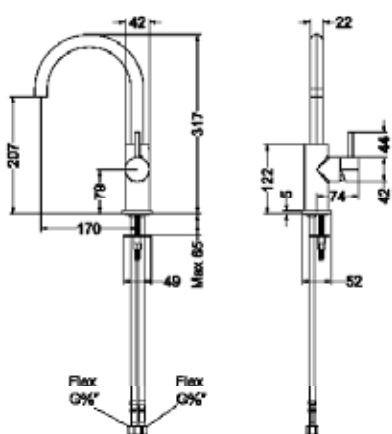
Wastafelmengkraan draaibare uitloop - Stilo
