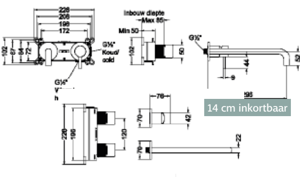
Inbouw wastafelkraan incl. inbouwbox - Stilo
