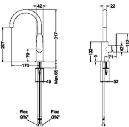
Wastafelmengkraan draaibare uitloop - Forma
