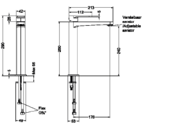
Wastafelmengkraan staand model L - Forma
