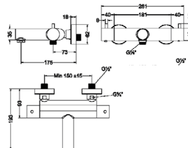
Opbouw badthermostaatkraan met vaste uitloop
