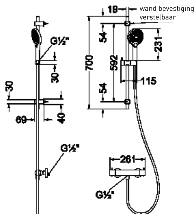
Douchethermostaat opbouw
